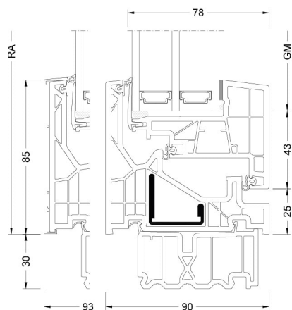
Senkrecht / Vertical
